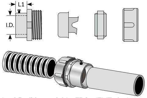
(Metal flexible conduit) EBG (EMT pipe)
