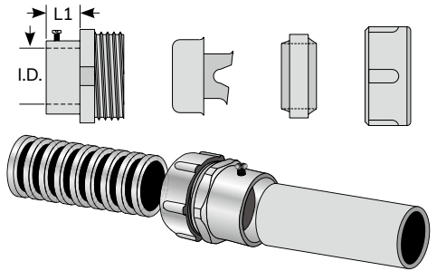
(Metal flexible conduit) PBG (PVC pipe)
